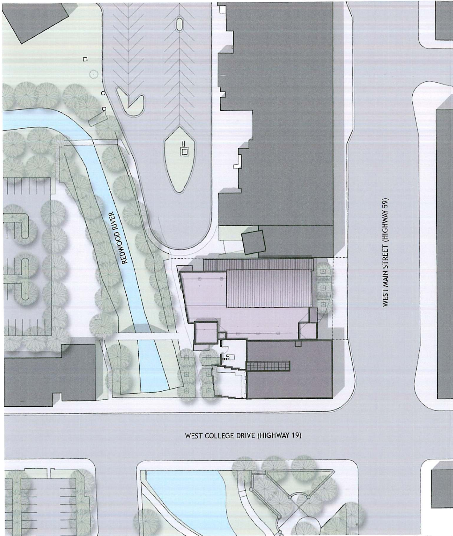
5 - SITE PLAN
